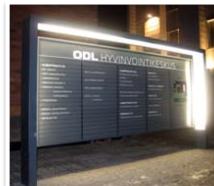
Valaistu ulko-opaste, teräsrunko, vaihdettavat alumiiniset tekstiprofiilit
